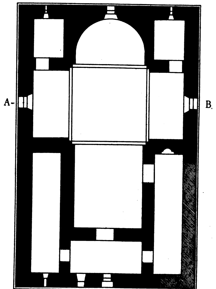
ПЛАНЪ ЦЕРКВИ ВЪ ДОЛИСЪ-ХАНЪ.
