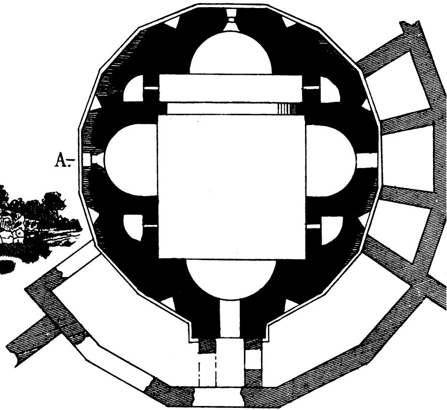
ПЛАНЪ ХРАМА ВЪ СВЕТИ.
