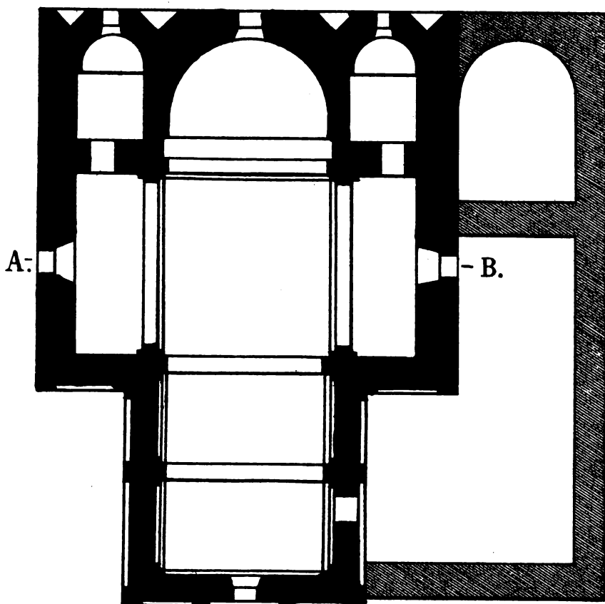
ПЛАНЪ ЦЕРКВИ ВЪ ЭНИРОБАТЪ.
