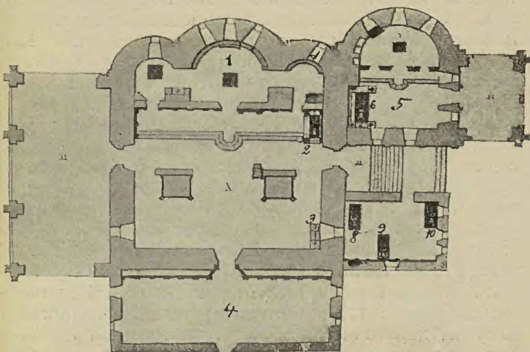
Планъ Троицкаго собора XVII вѣка.
