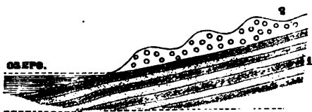
Разрѣзъ новѣйшихъ формаций у Иссык-куля.
