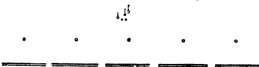
Черт. № 23 Полкъ въ линіи (т. е. въ развернутомъ строю)
