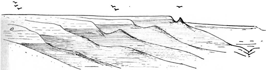
Рис. 16. Край Устюрта, обращенный къ Джанаку. Три птички обозначаютъ Кіа-джоль, двѣ — Кумчоку, а одна — Карамурунь.
